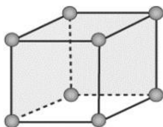
Simple cubic
