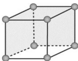
Simple cubic
